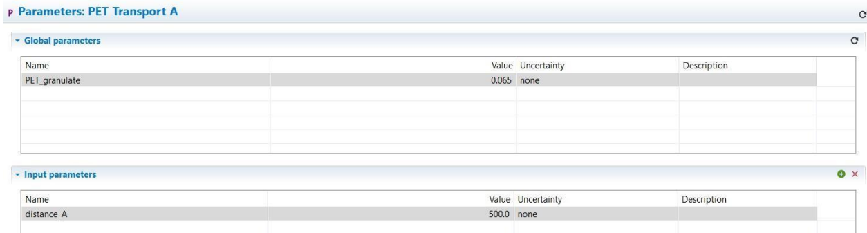
Figure 8.5: Parameters tab
